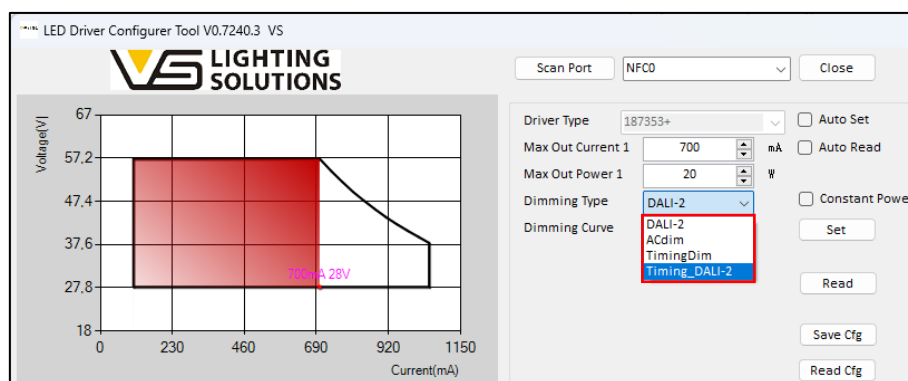
Abbildung 20 – Auswahl des Dimmtyps (Primeline NFC S-MD DALI2 Dx)
