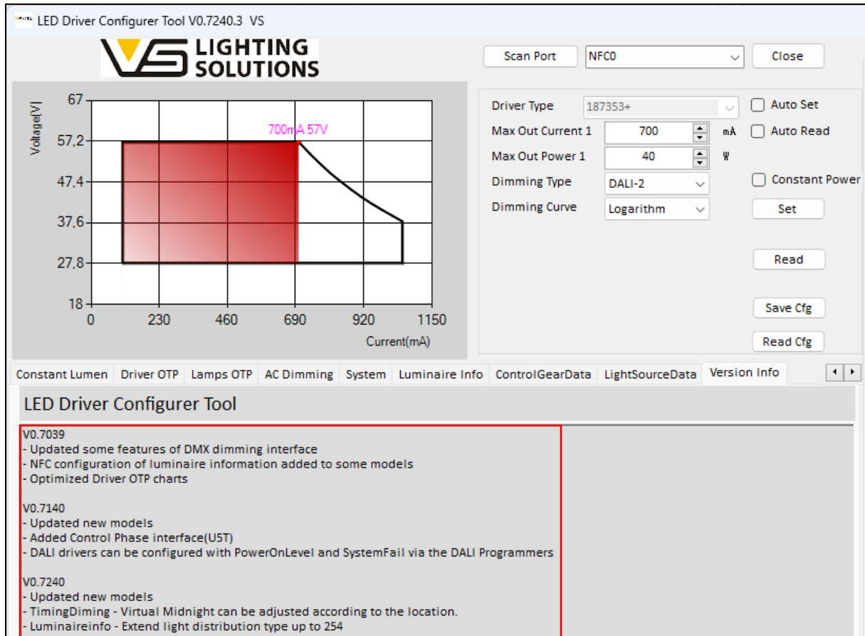
Abbildung 46 – Software-Version und Change Log
