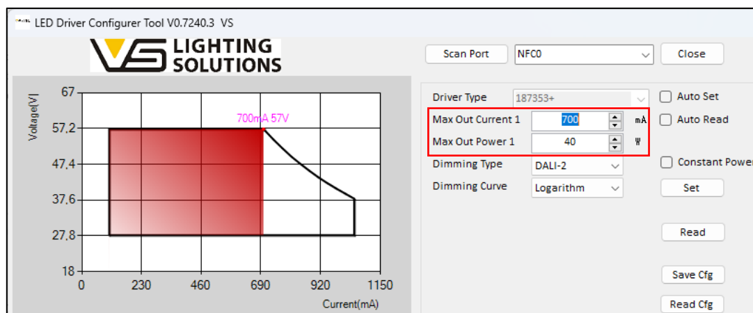
Abbildung 19 – Einstellung des Ausgangsstroms
