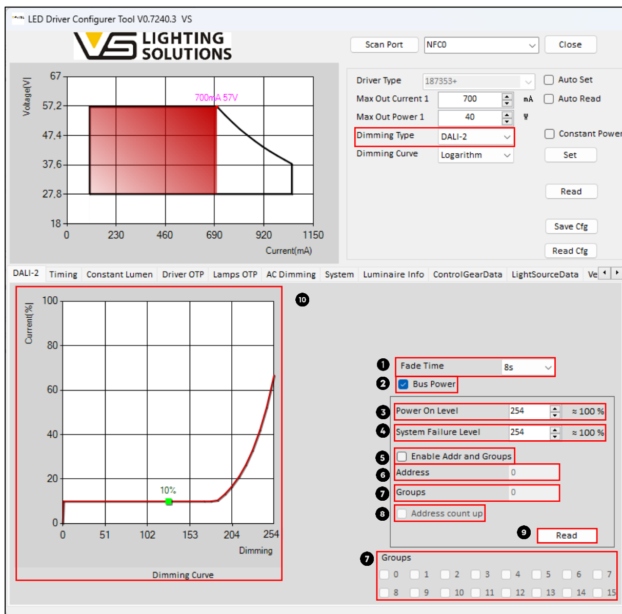
Abbildung 23 – DALI2-Dimmung Konfiguration
